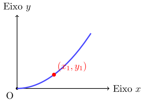
Figura 1.4: Gráfico de coordenadas cartesianas.
